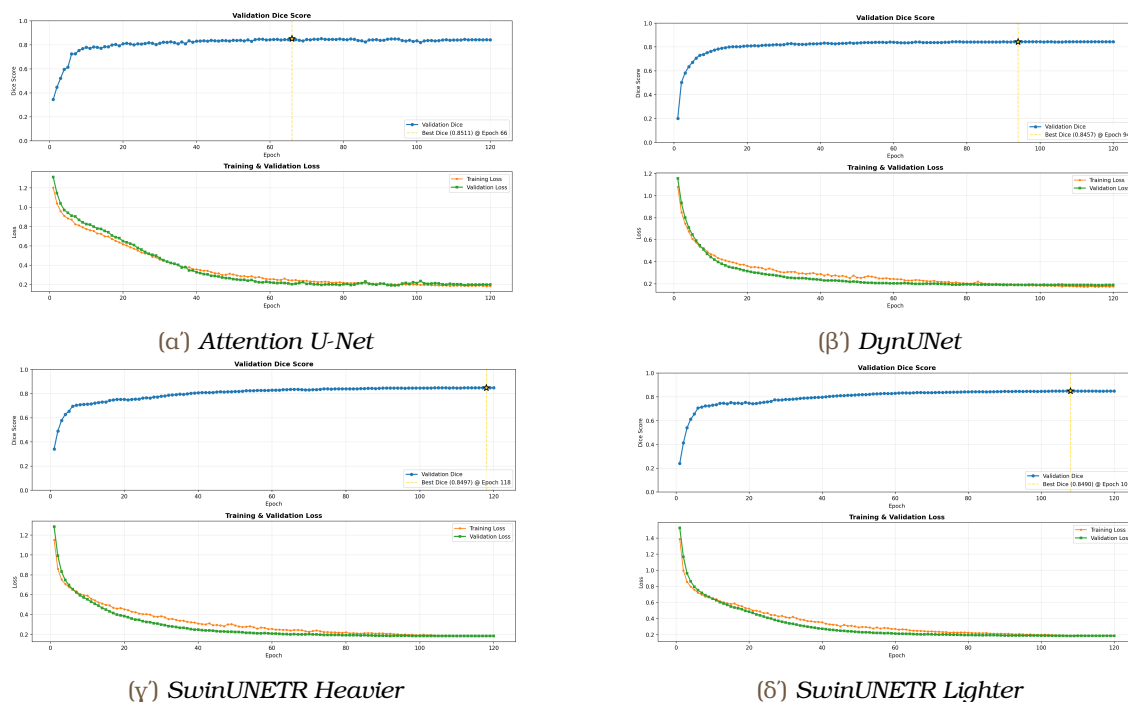
Εικόνα 6.1: Καμπύλες εκπαίδευσης: Validation Dice (πάνω) και training/validation loss (κάτω) για Attention U-Net, DynUNet, SwinUNETR Heavier και SwinUNETR Lighter. Το \sigma τέρι και η κατακόρυφη διακεκομμένη γραμμή δείχνουν το epoch του καλλίτερου Dice.
