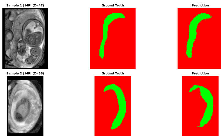
Εικόνα 6.10: U-Net
